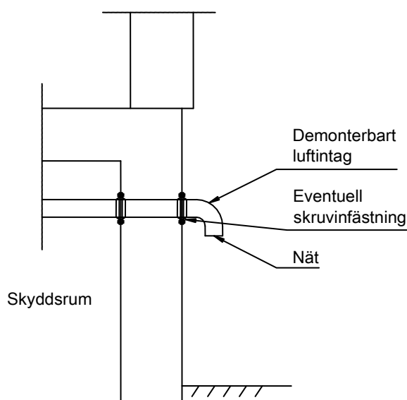
Figur T23-101e. Alternativt utförande av utvändigt luftintag.
