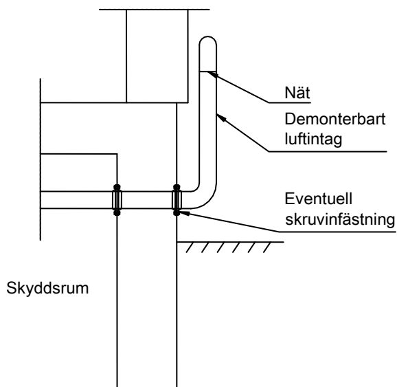
Figur T23-101d. Alternativt utförande av utvändigt luftintag.
